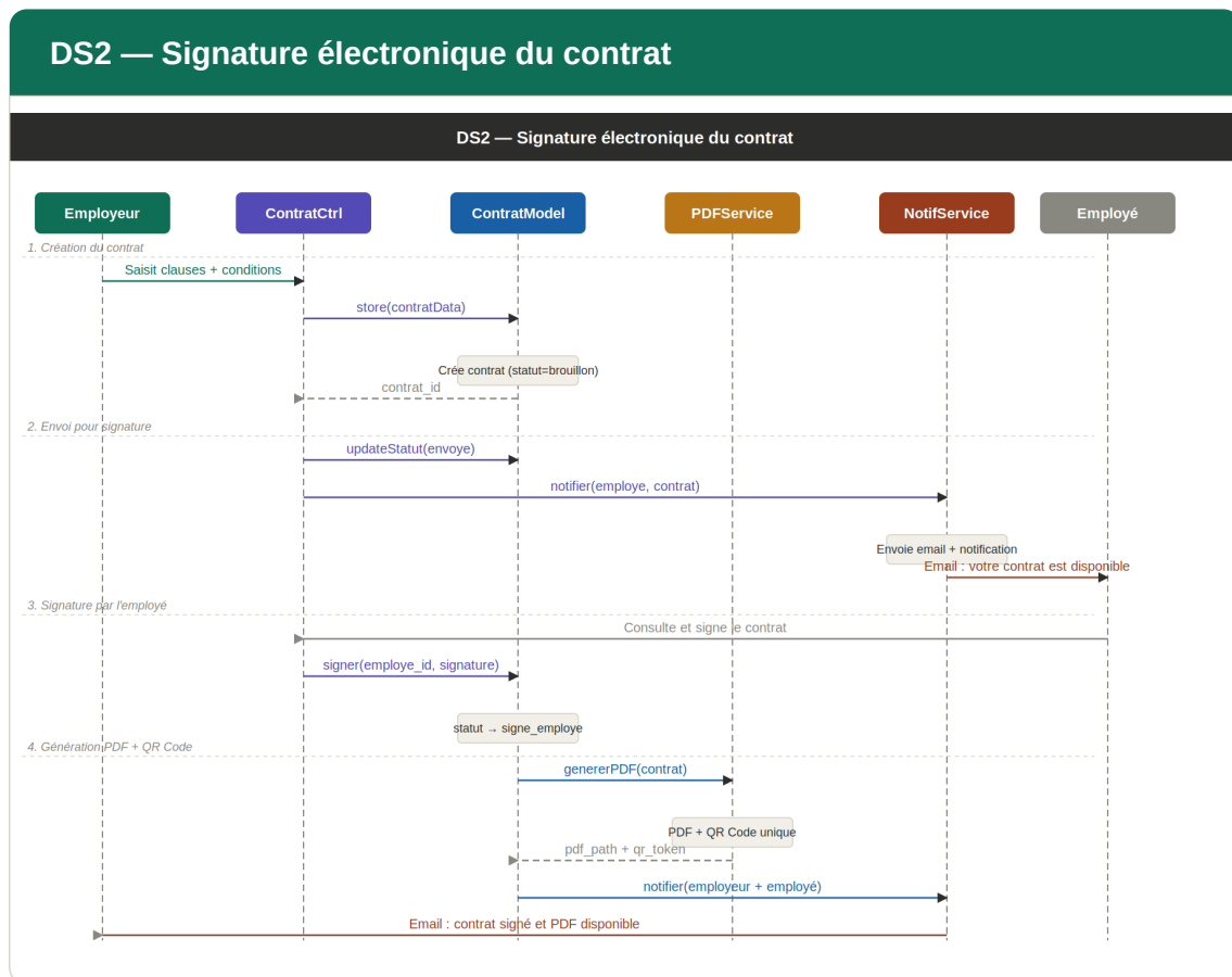
Figure 6 — DS2 : Signature du contrat · Acteurs : 6 composants · Étapes : 12 messages
