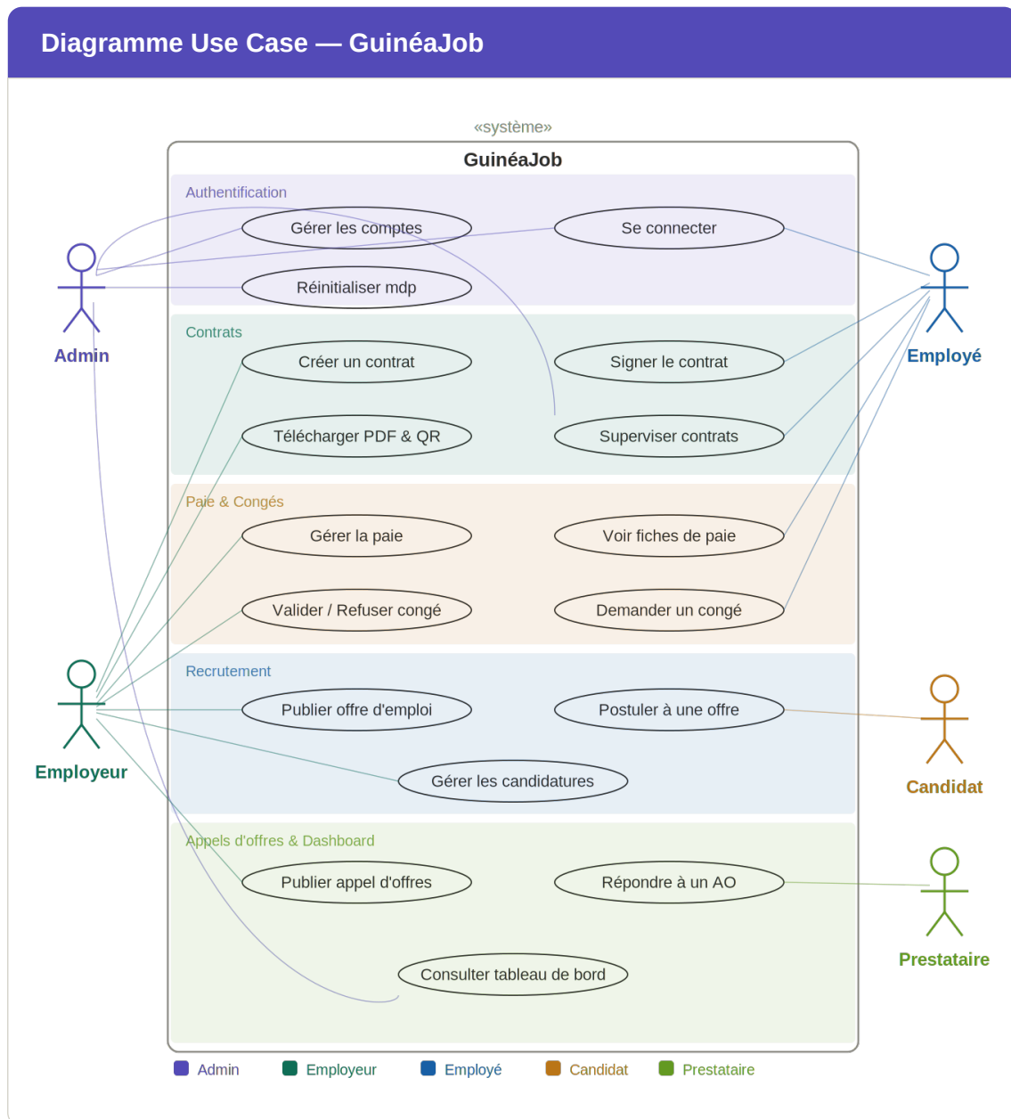
Figure 3 — Diagramme des cas d'utilisation UML · GuinéeJob v1.1
