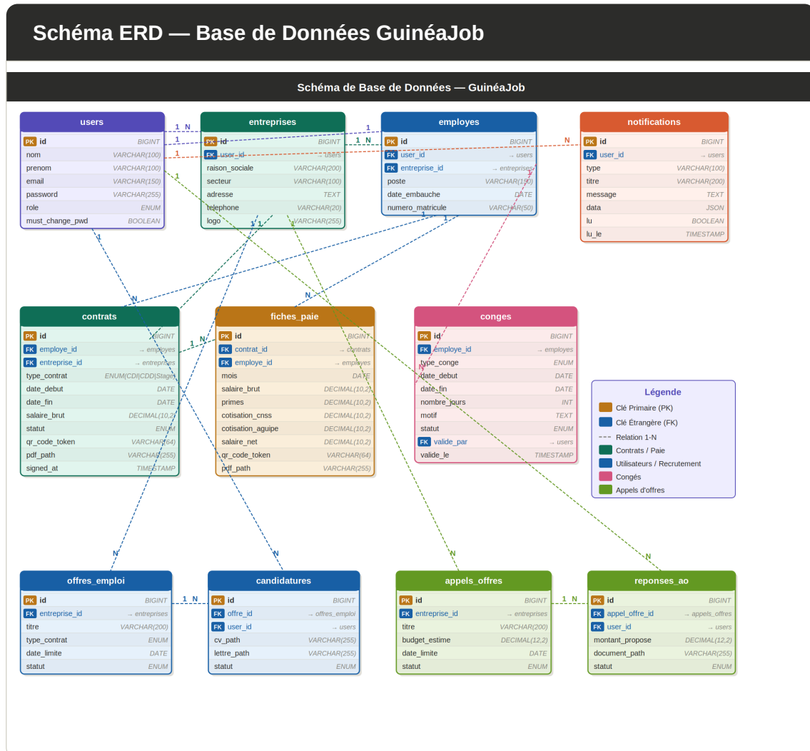
Figure 2 — Schéma ERD · GuinéeJob v1.1 · 11 tables · 101 champs · 15 relations
